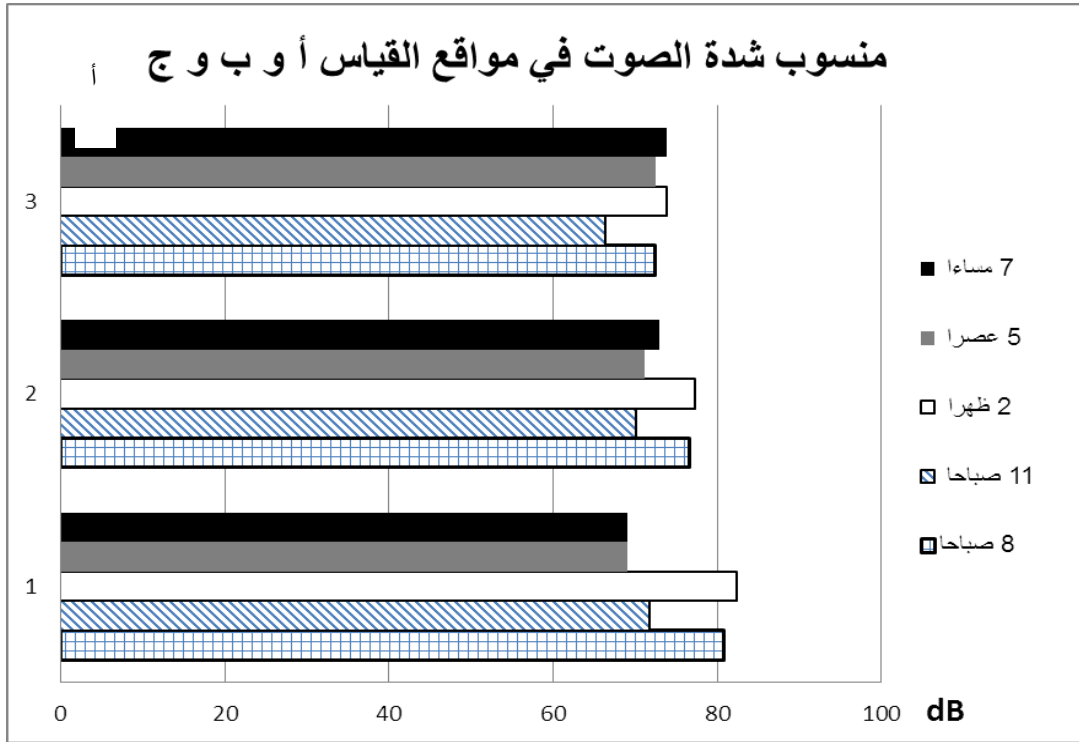
الشكل (٥): يوضح منسوب شدة الصوت المسجلة في مواقع القياسات (أ) و(ب) و(ج) وفي اوقات متنوعة من اليوم/ اعداد الباحث
