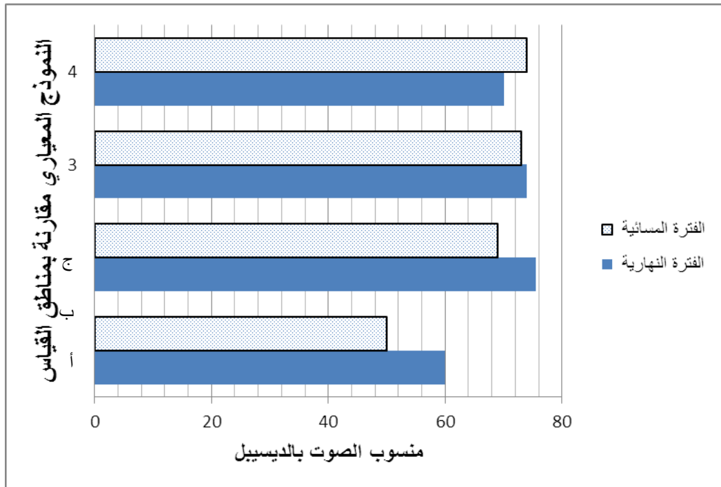
الشكل (٦): يوضح مناسيب شدة الصوت المسجلة في مواقع القياسات (أ) و(ب) و(ج) ومقارنتها بالنموذج المعياري لمناسيب الصوت المعتمدة عالميا/ اعداد الباحث
