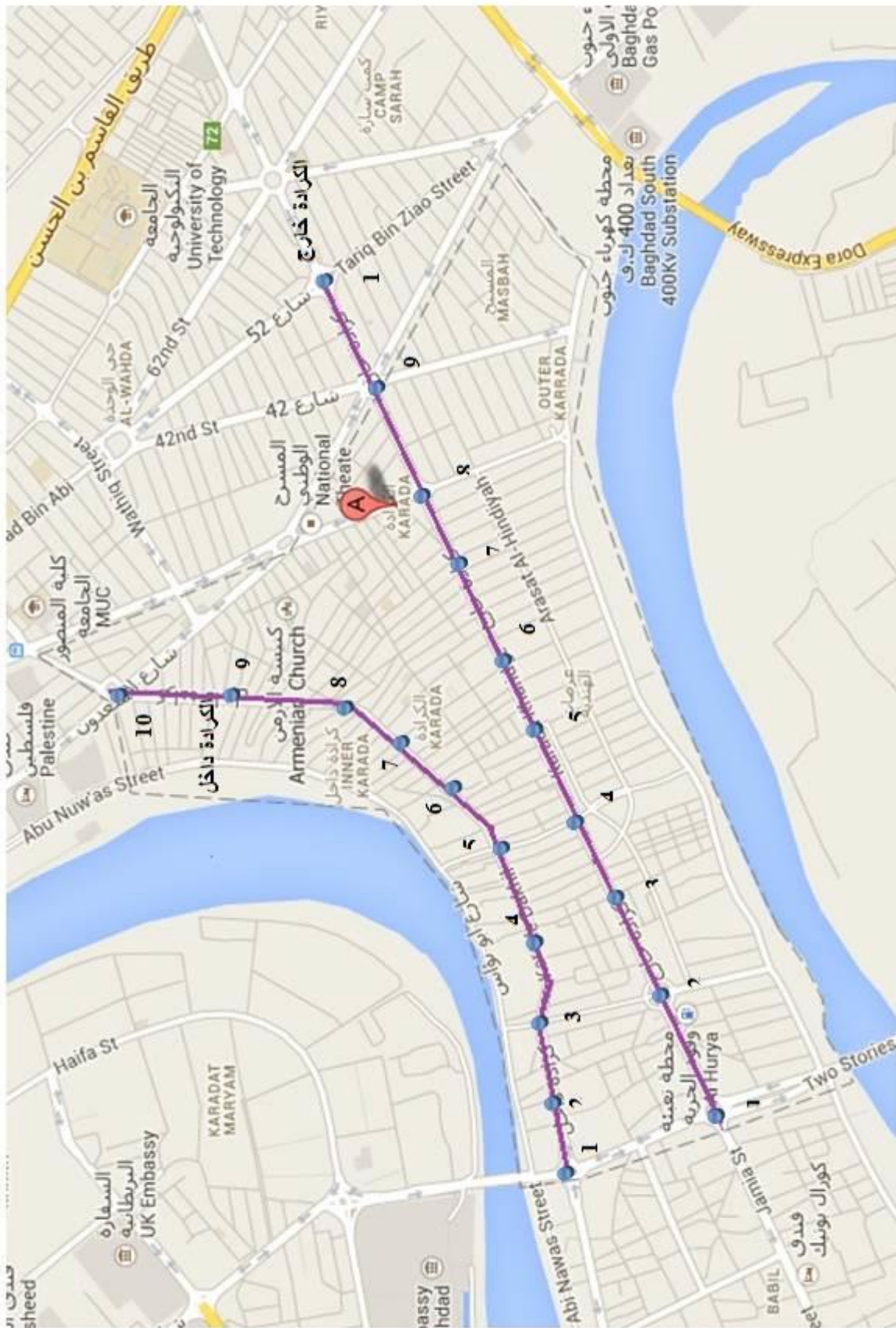
الشكل (10) مواقع قياسات مناسب شدة الاصوات في الشوارع الرئيسية لمنطقة الكرادة / اعداد الباحث
