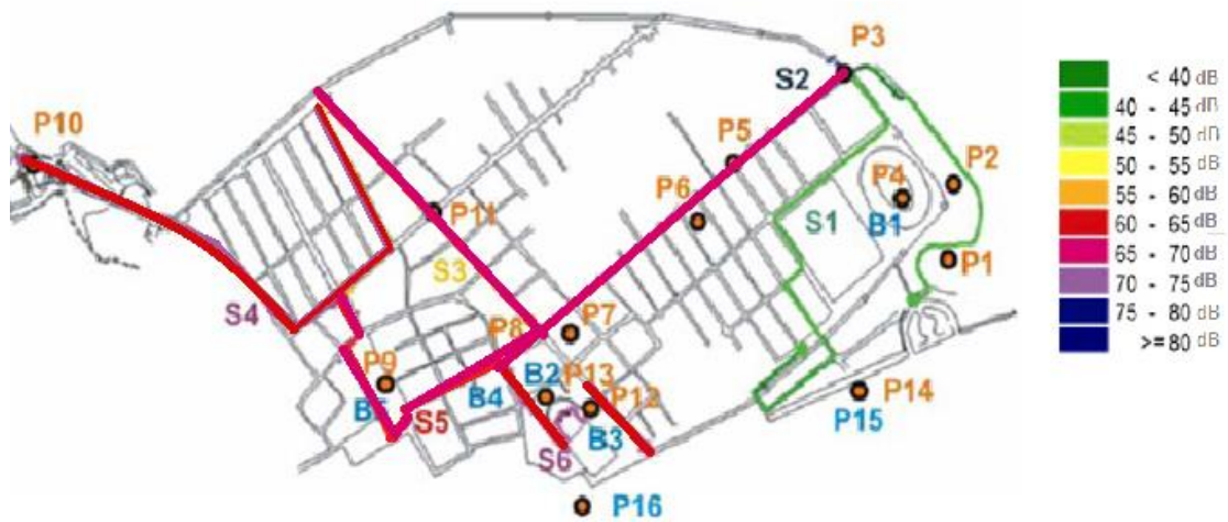
الشكل (٣): مخطط المنطقة المنتخبة للدراسة في مدينة بومباي وعليها اماكن القياسات الصوتية وحركة المشاة وفق مفتاح مناسيب الصوت [١٦]
